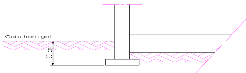
Profondeur d'ancrage des fondations
