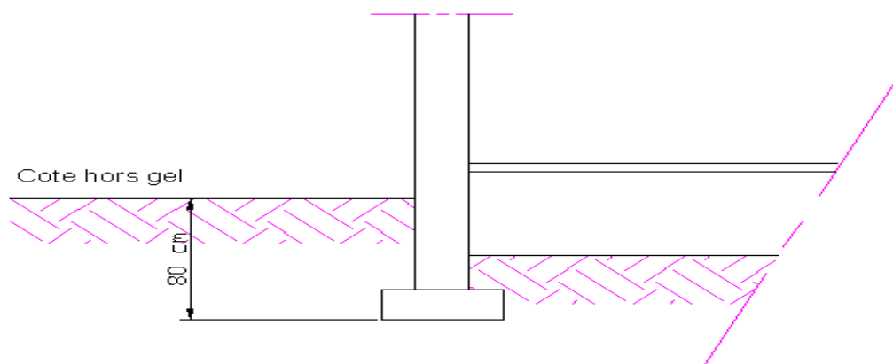
Profondeur d'ancrage des fondations
